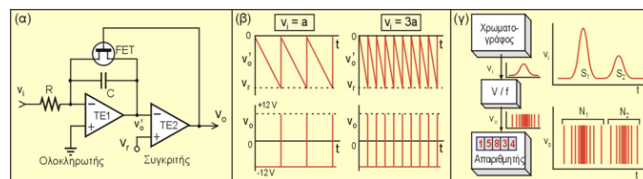
Σχήμα 2. (α) Κύκλωμα μετατροπέα V/f με δύο τελεστικούς ενισχυτές. (β) Οι κυματομορφές των τάσεων v_o' και v_o (ενδεικτικά για δύο διαφορετικές τάσεις σήματος εισόδου v_i = a και v_i = 3a ). (γ) Τυπική σύνδεση της εισόδου μετατροπέα V/f με το σήμα του ανιχνευτή αεριοχρωματογράφου. Για κάθε χρωματογραφική κορυφή, οι παλμοί εξόδου του μετατροπέα V/f απαριθμούνται με ψηφιακό απαριθμητή και ο αριθμός τους είναι ανάλογος του ολοκληρώματος (επιφάνειας) της κάθε κορυφής ( N_i = k S_i ).
