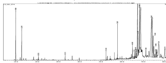
Χρωματογράφημα 1. μαστίχα Χίου μετά από εκχύλιση σε αηθκολικό διάλυμα
