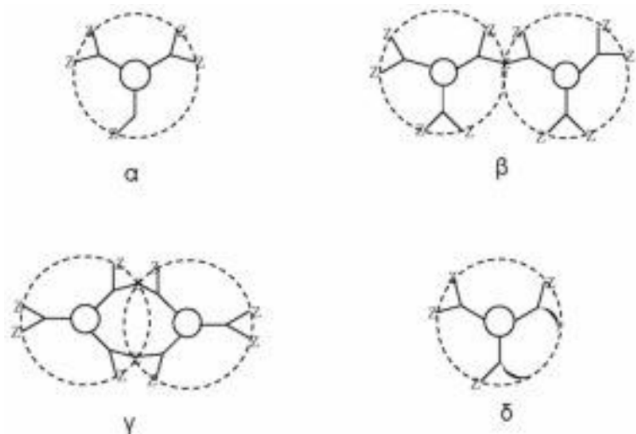
Σχήμα 4:Απεικόνιση των εξής ατελειών α) έλλειψη κλάδου, β), γ) διαμοριακή σύζευξη κλάδων, δ) ενδομοριακή σύζευξη κλάδου.
