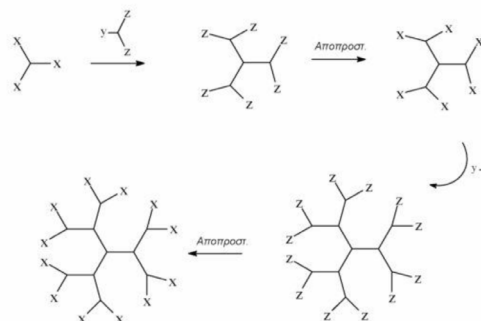
Σχήμα 3: Αναπαράσταση της αποκλίνουσας μεθόδου σύνθεσης ενός Δενδριμερούς
